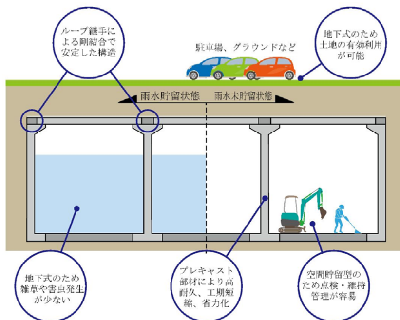
図 2.1-3 アクアポンドL型工法の特長
