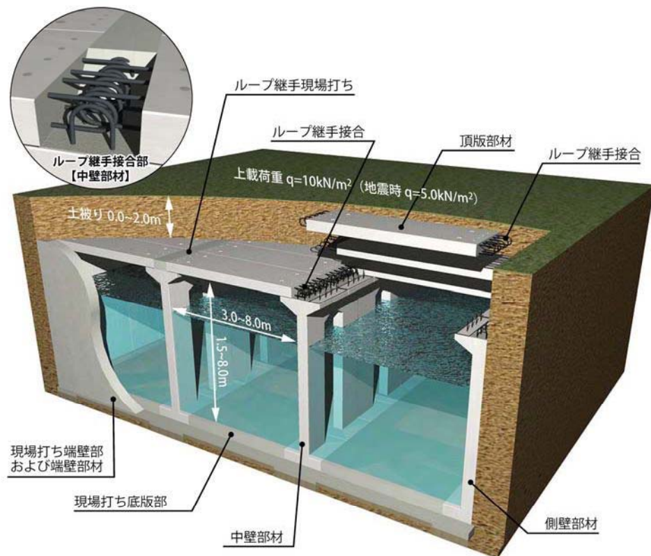
図 1-1 アクアポンドL型工法の概要図
